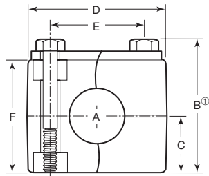
Einzel-Schelleneinheit
